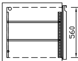
GN-Auflageschienen mit Stellschienen Best.-Nr.: 3500-GN
